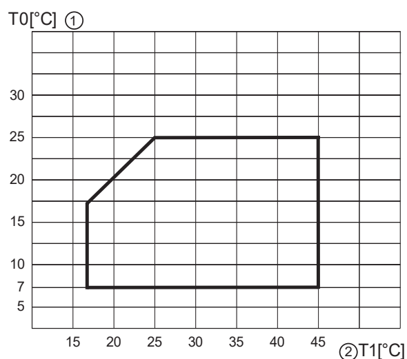
Einsatzgrenzen Kühlen
