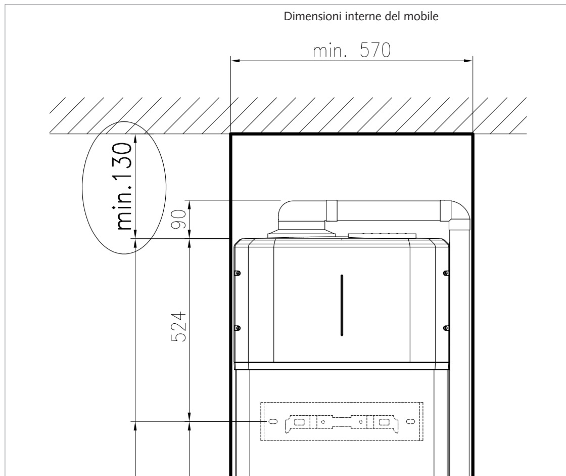
Fig.: Distanza minima dal soffitto
