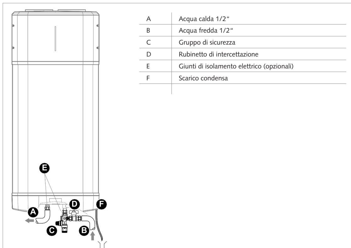
Fig.: Collegamenti idraulici
