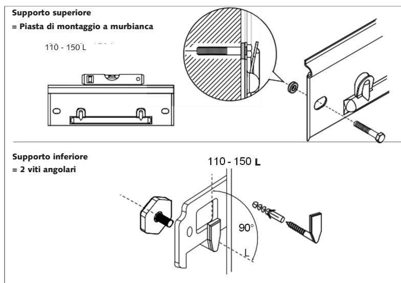
Fig.: Montaggio a parete
