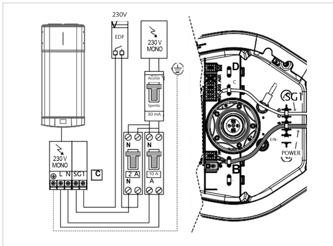
Fig.: Collegamento elettrico (segnale HC-HP)
