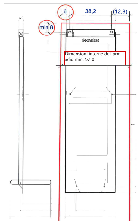
Fig.: Staffa orientabile a parete Dimensioni di montaggio
