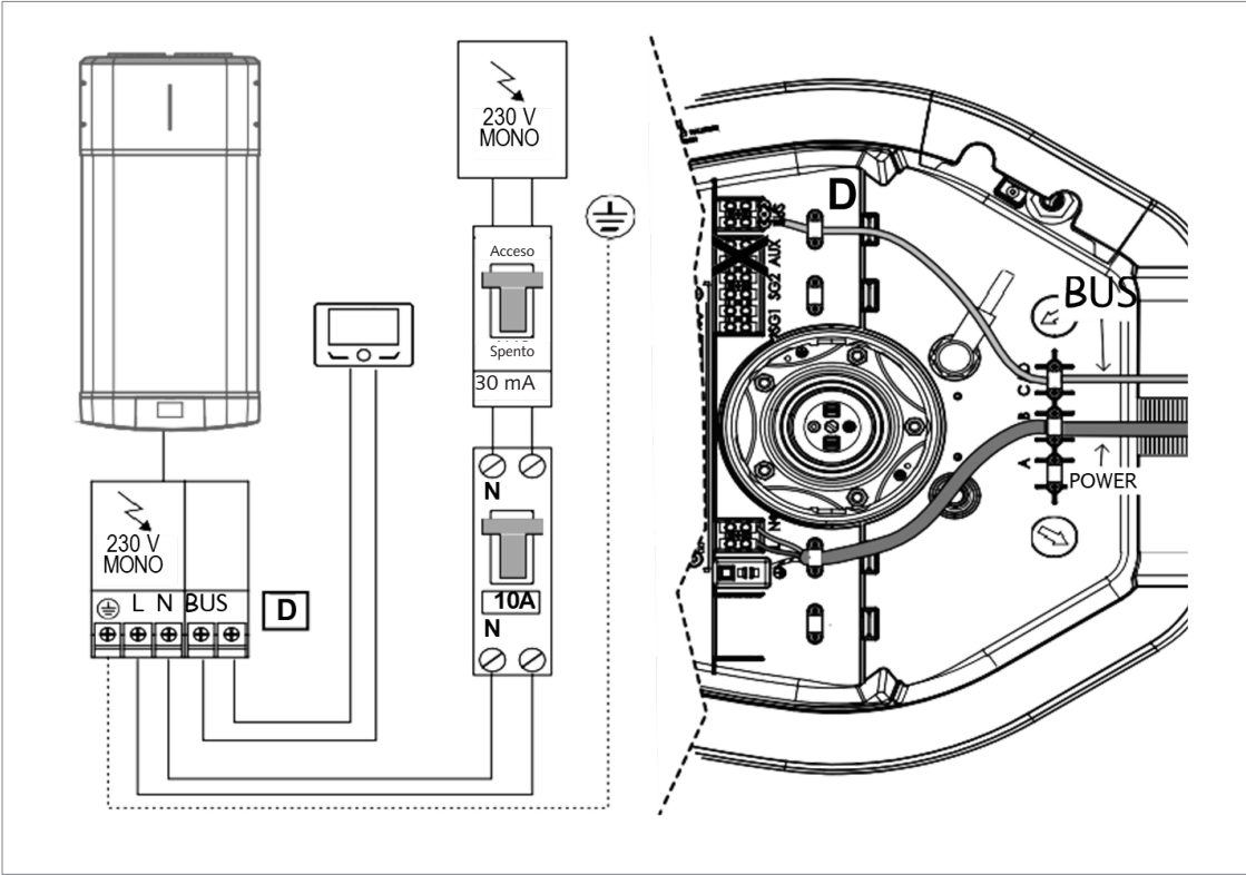
Fig.: Collegamento BUS
