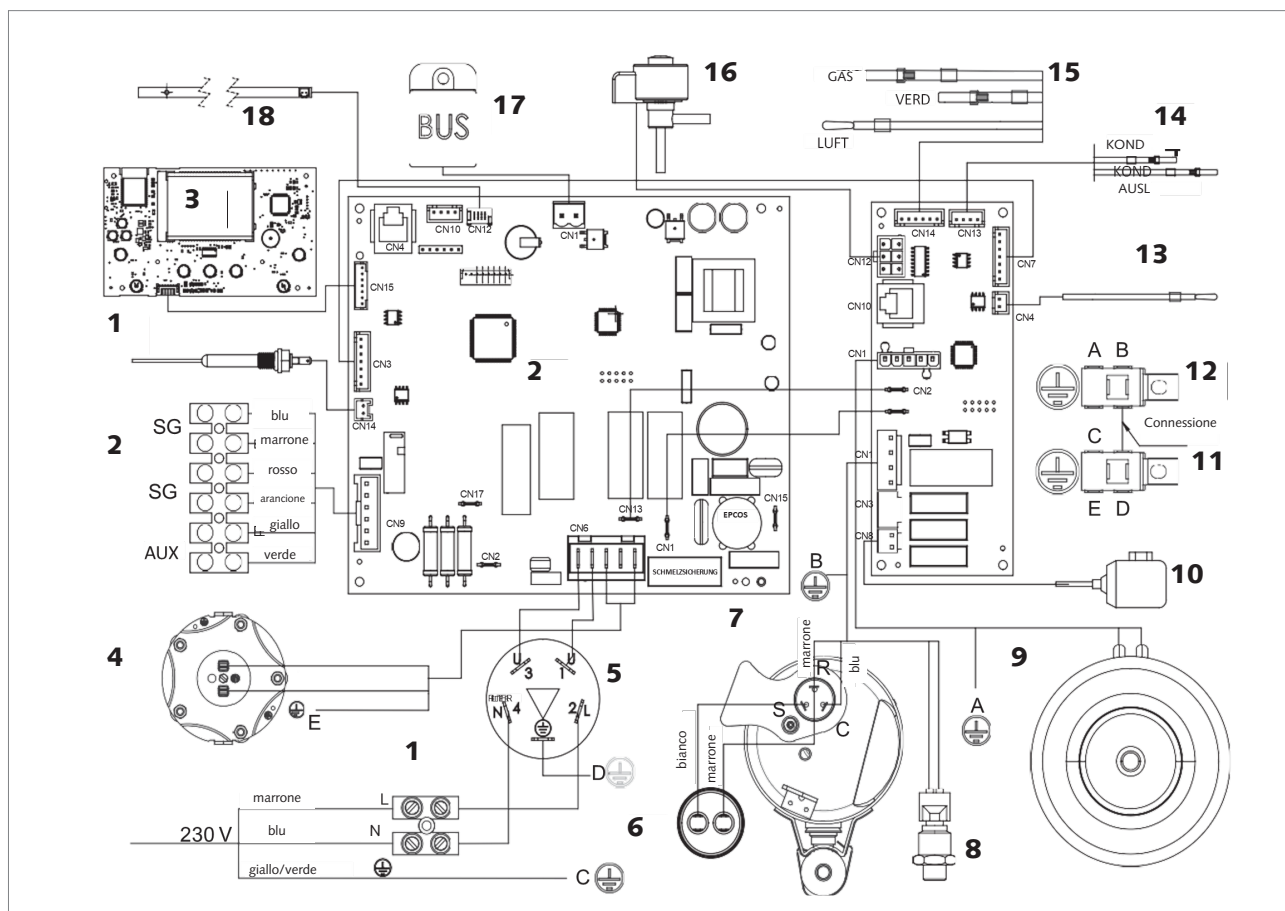
Fig.: Schema elettrico
