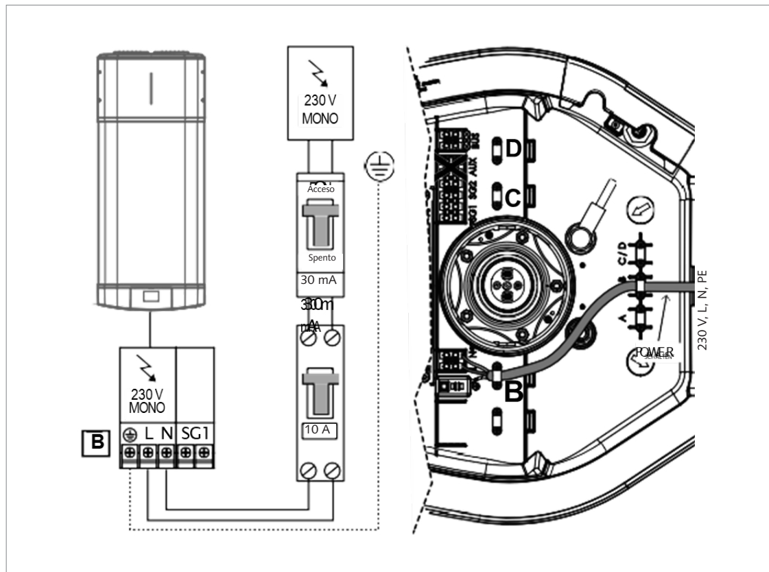
Fig.: Collegamento elettrico permanentess
