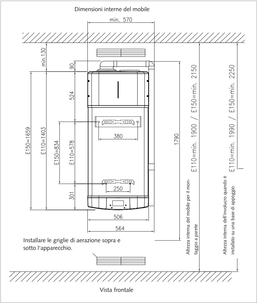
Fig.: Dimensioni
