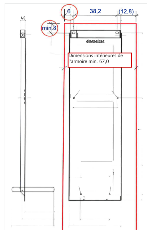
III. : Support mural pivotant Dimensions de montage
