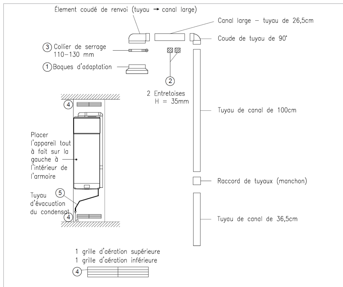
III. : Instructions de montage du conduit d'évacuation
