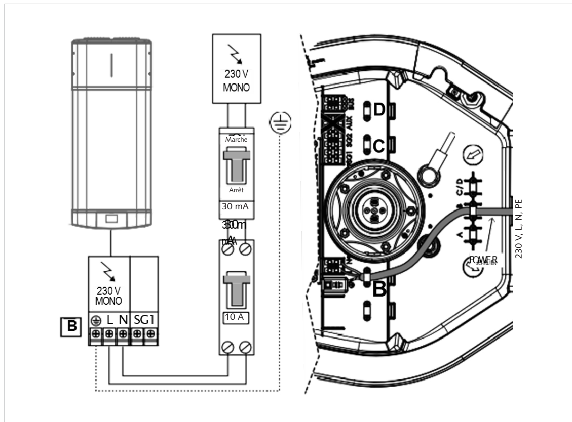
III. : Raccordement électrique permanent
