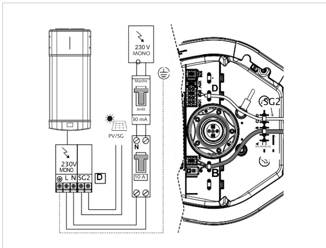
III. : PV ou SMART GRID (SG2)
