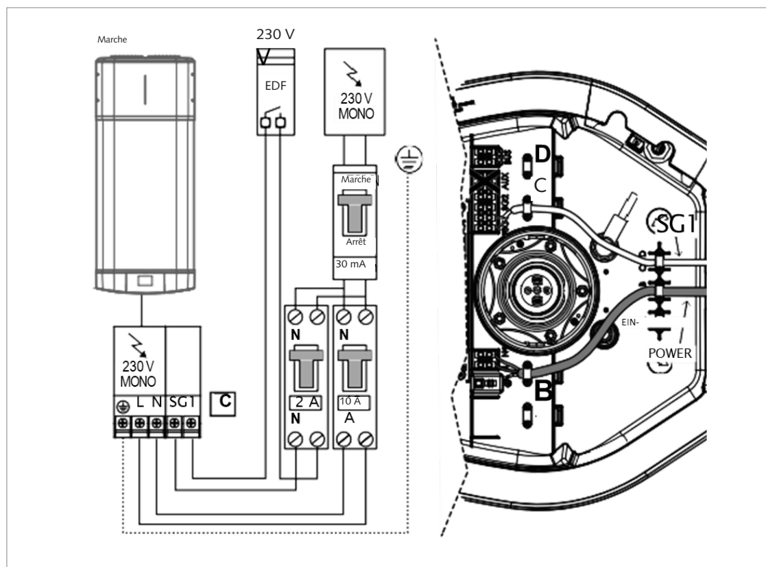
III. : Raccordement électrique avec tarif bi-horaire et signal HC-HP
