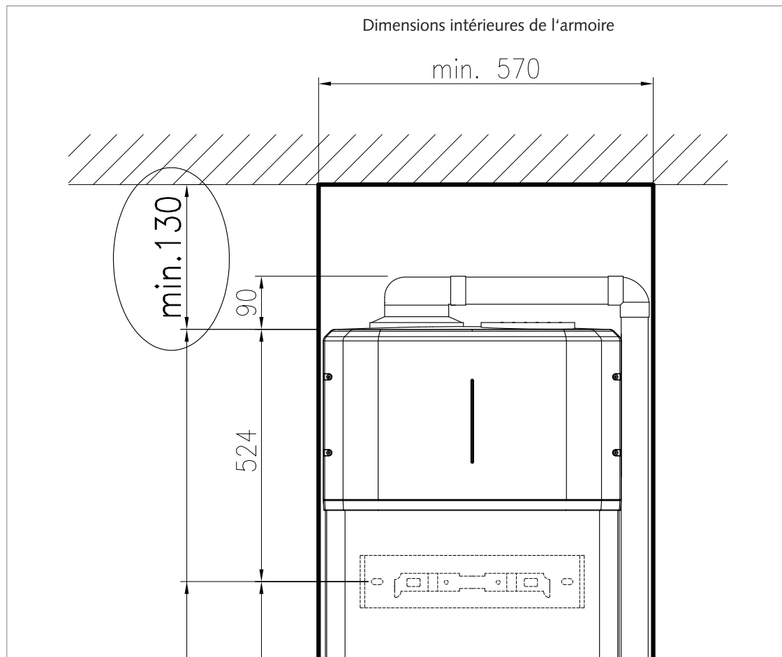
III. : Distance minimale au plafond
