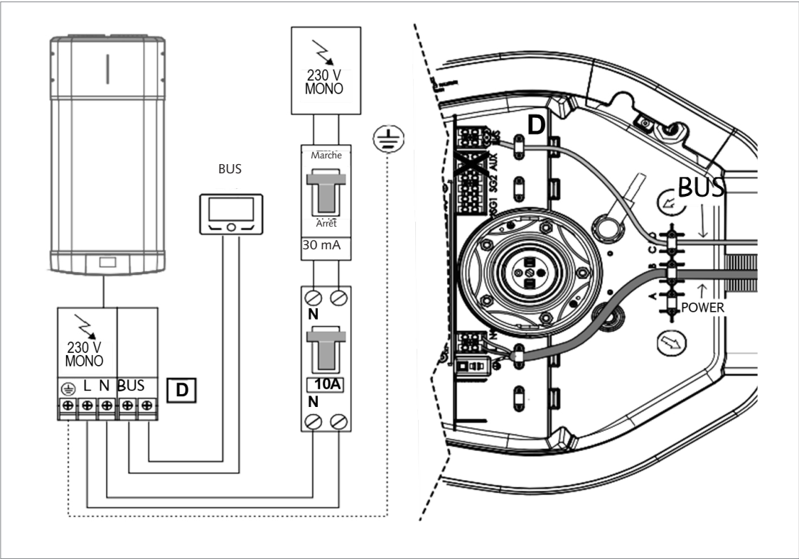
III. : Connexion BUS
