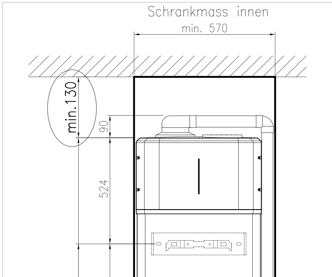
Abb.: Minimaler Deckenabstand
