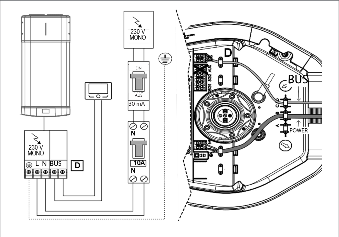
Abb.: BUS-Anschluss
