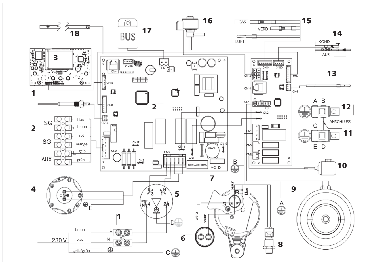
Abb.: Elektroschema
