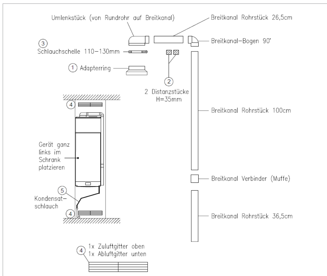
Abb.: Montageanleitung Abluftrohrkanal
