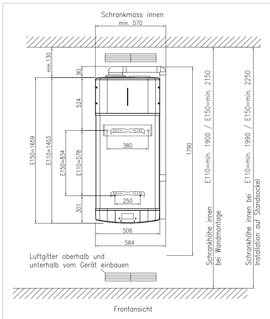
Abb.: Abmessungen
