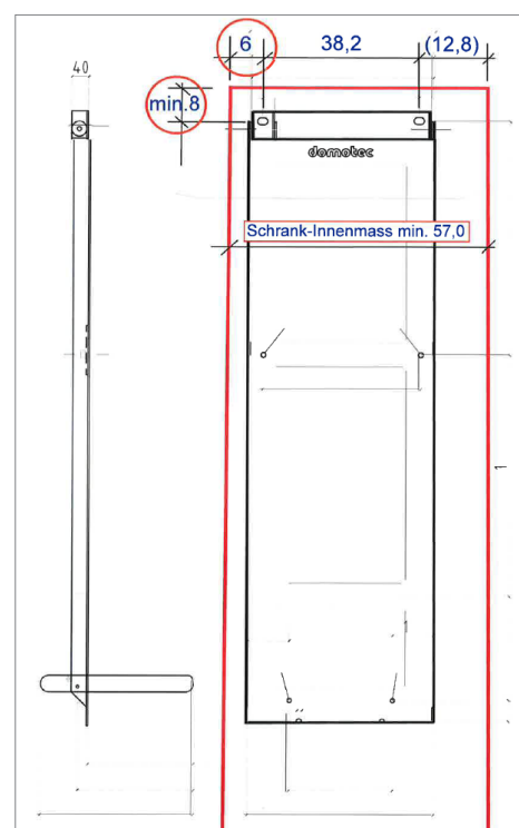
Abb.: Wandschwenkhalterung Montagemasse
