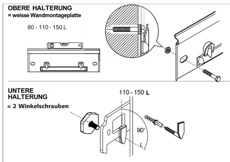
Abb.: Wandmontage
