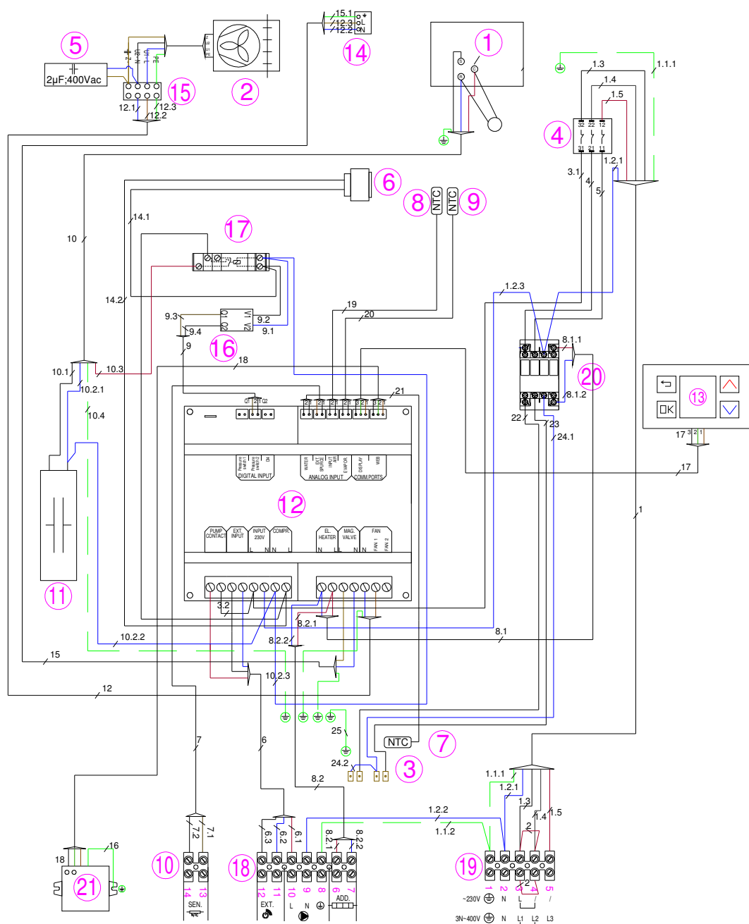
Abbildung 15: Elektrischer Schaltplan
