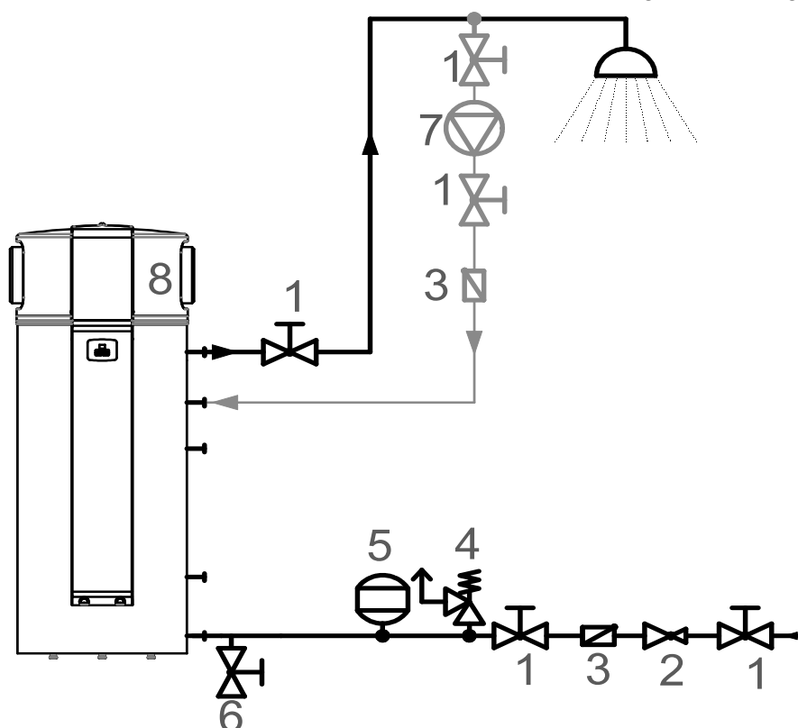
Abbildung 7: Anschluss ans Wasserversorgungsnetzwerk
